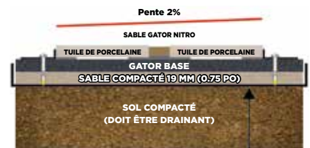
Option 3a • Tuiles de porcelaine sur Gator Base
