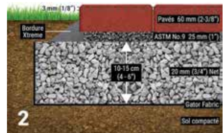
Option 2 • Perméable ou Hybride
